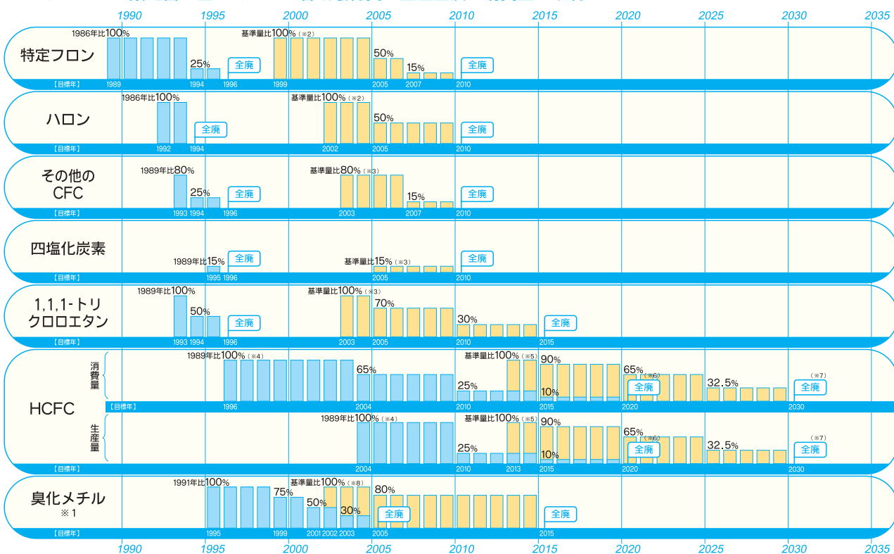
モントリオール議定書に基づくオゾン層破壊物質の生産量及び消費量の規制スケジュール
